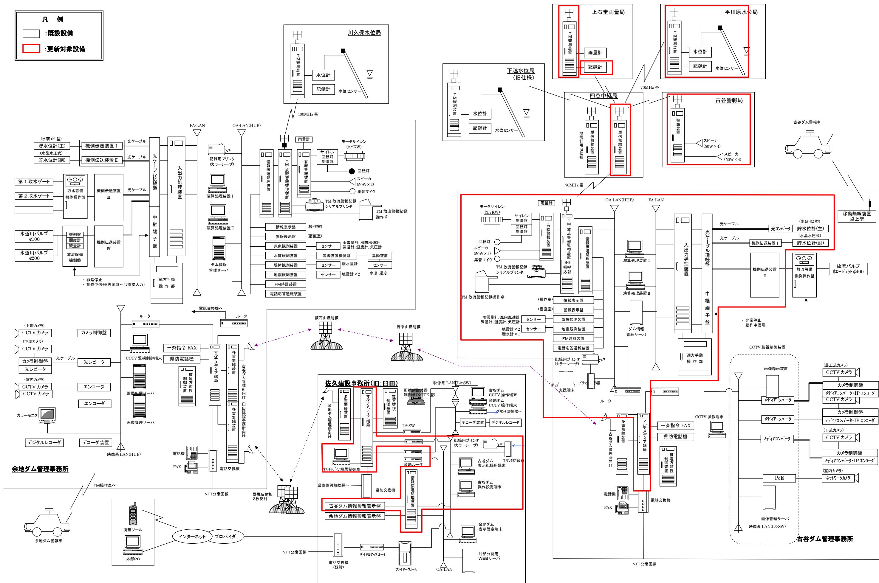
別図—1 システム全体構成図(ダムコン・気象観測・放流警報テレメータ更新対象) 古谷ダム
