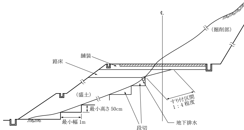
図 1-3-2 盛土基礎地盤の段切
