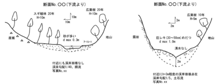
図 9-2-7 横断スケッチの例
