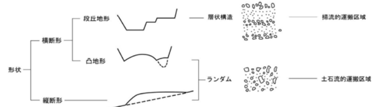
図 9-2-6 溪床土砂堆積地の形状及び断面の粒径の配列による分類
