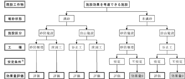
図 9-2-4 横断構造物の施設効果量の評価
