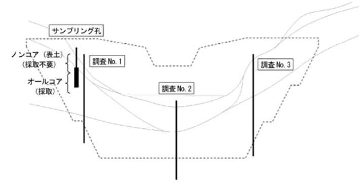
図 9-2-16 サンプルング位置の選定
