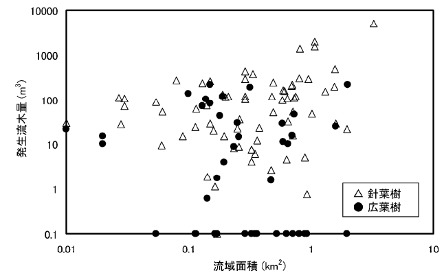
図 9-2-13 流域面積と発生流木量
