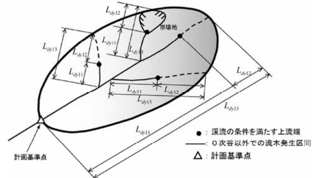
図 9-2-12 流木発生区間長さ
