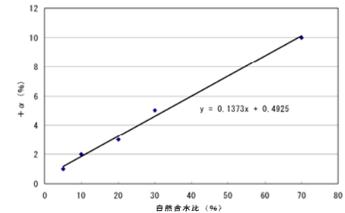
図 9-2-17 自然含水比と加水量（加水側含水比）の経験式
