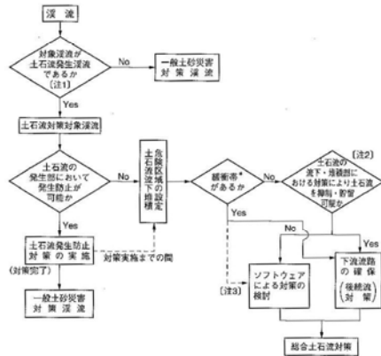
図4.2 総合土石流対策の基本的考え方
