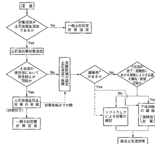
図 9-1-21 総合土石流対策の基本的考え方
