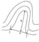
図2-1 1次谷
