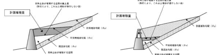
図 9-1-15 計画堆積土砂量の考え方
