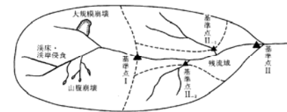
図 9-1-2 砂防基本計画系統図
