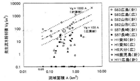
図-2 流域面積と発生流木幹材積
