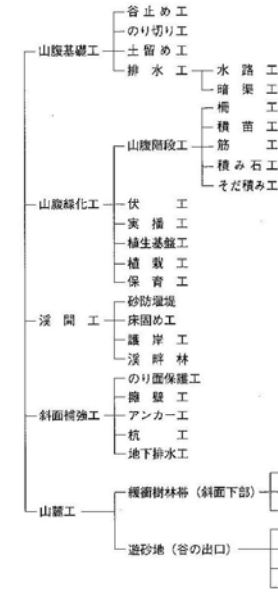
図 9-1-24 都市山麓グリーンベルトの整備に用いられる主な工法
