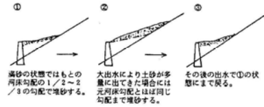
図 3.3.7 (b) 不透過型砂防堰堤の調節量
