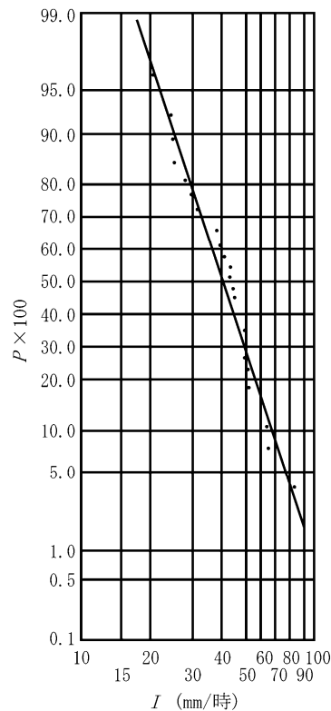
図2.5.4 確率降雨算定図
