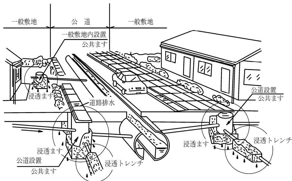
図2.5.6 下水道雨水浸透施設の概念図
