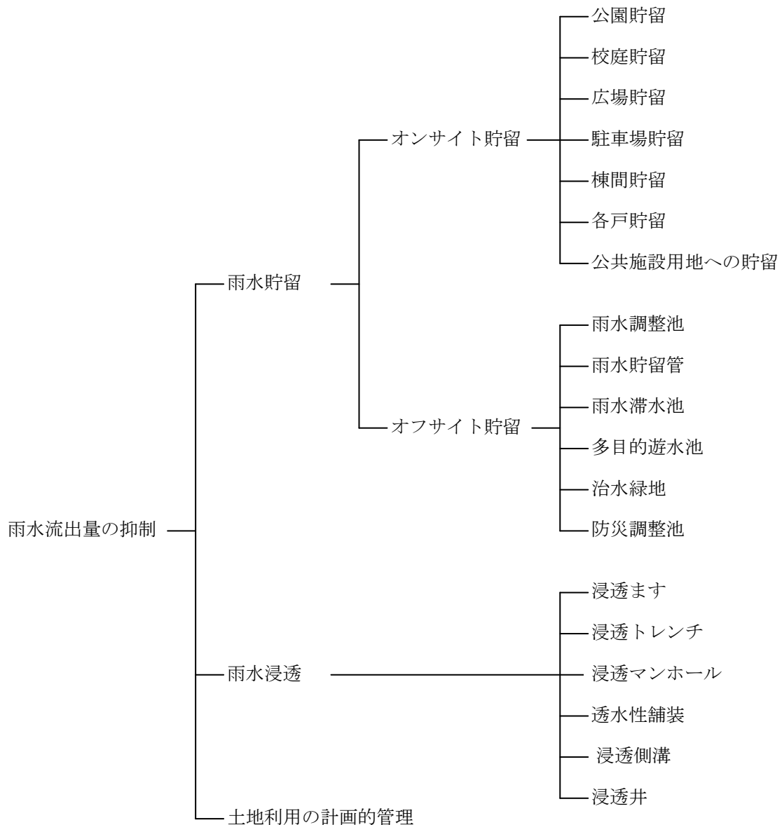
図2.5.5 雨水流出量の抑制方法の分類
