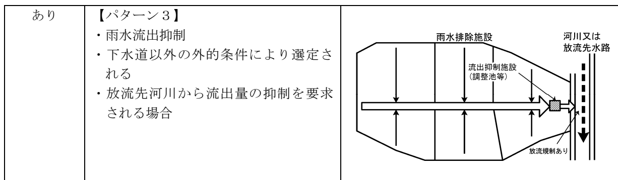
図2.5.1 雨水管理計画策定における整備手法例
