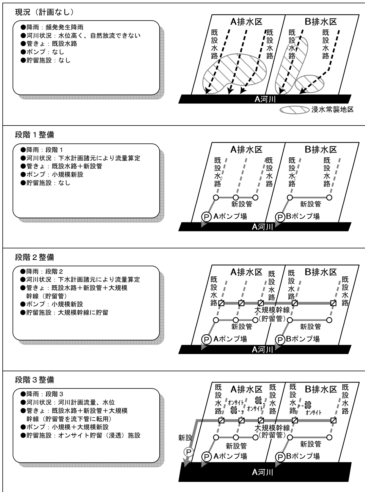
図2.5.7 雨水排除施設の段階的整備（例）
