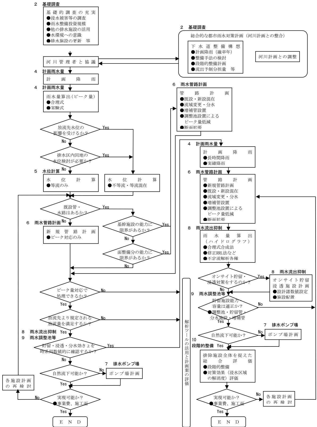
図2.5.2 雨水排除計画策定フローチャート
