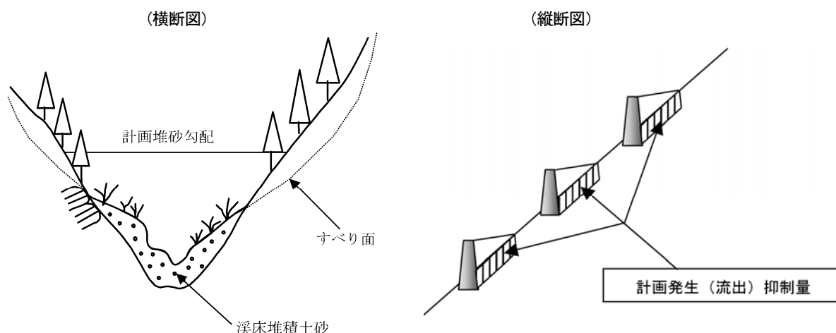
図 9-3-5 溪床堆積土砂移動防止工の計画で扱う土砂・流木量等のイメージ
