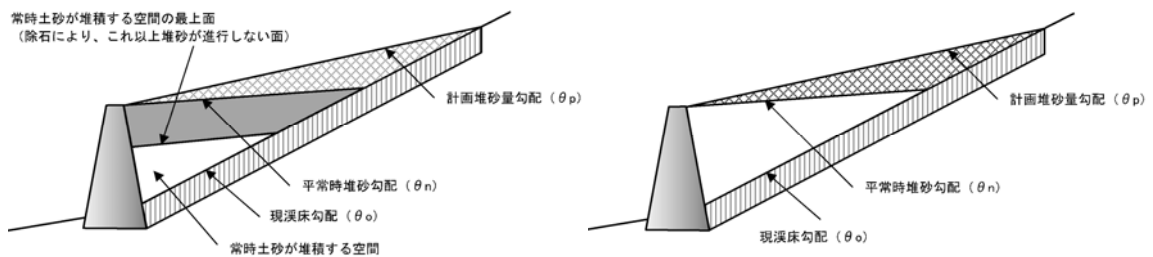
図 9-3-4 砂防堰堤の型式別の計画で扱う土砂・流木量等の模式縦断面図
