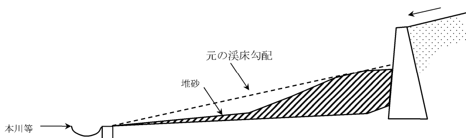
図 9-3-8 土石流堆積流路のイメージ
