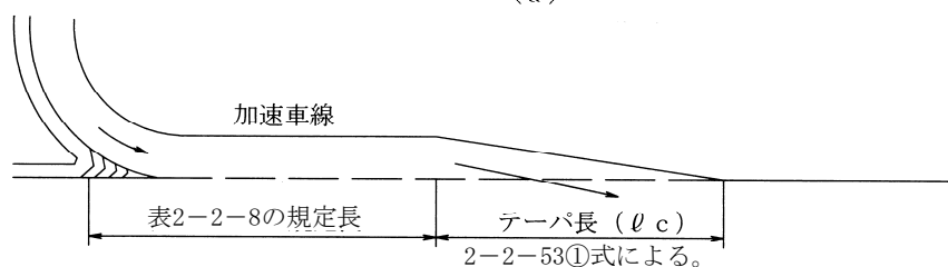
図 2-2-24 変速車線長
