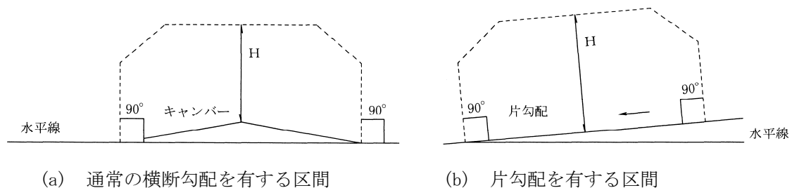
図 2-2-8 建築限界線のとり方
