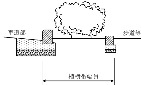
図2-2-12 植樹帯断面の例
