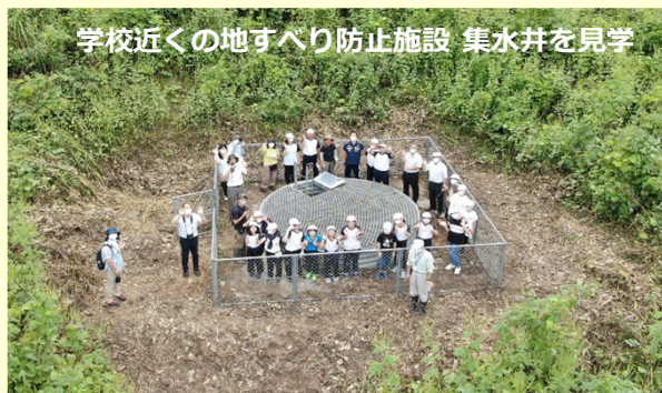
地下水が集水井に集まる様子を見ている
