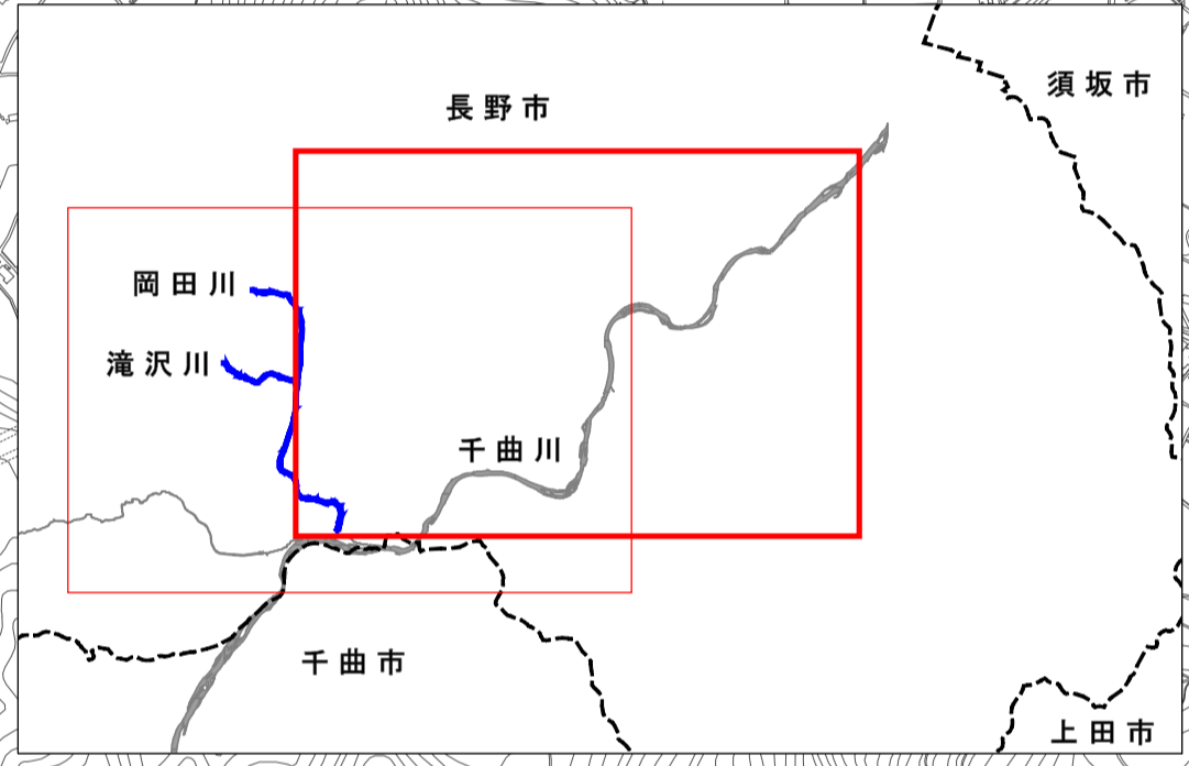
信濃川水系 岡田川、滝沢川 洪水浸水想定区域図 (想定最大規模降雨)
