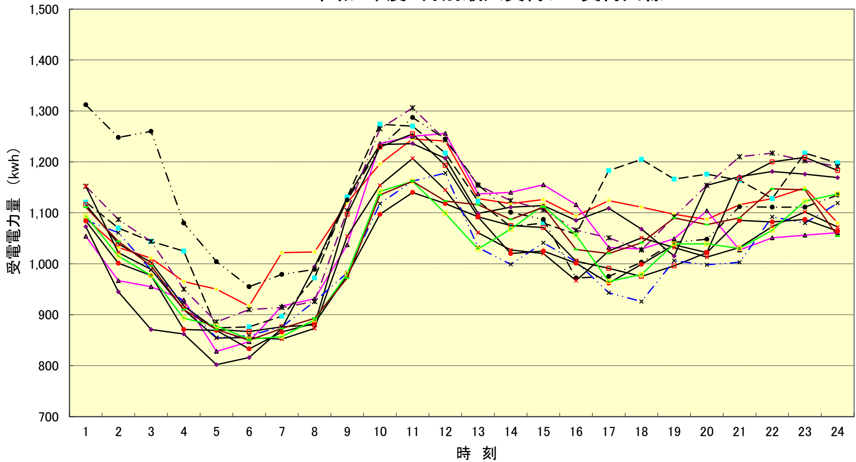
令和4年度 月別最大負荷日 負荷曲線
