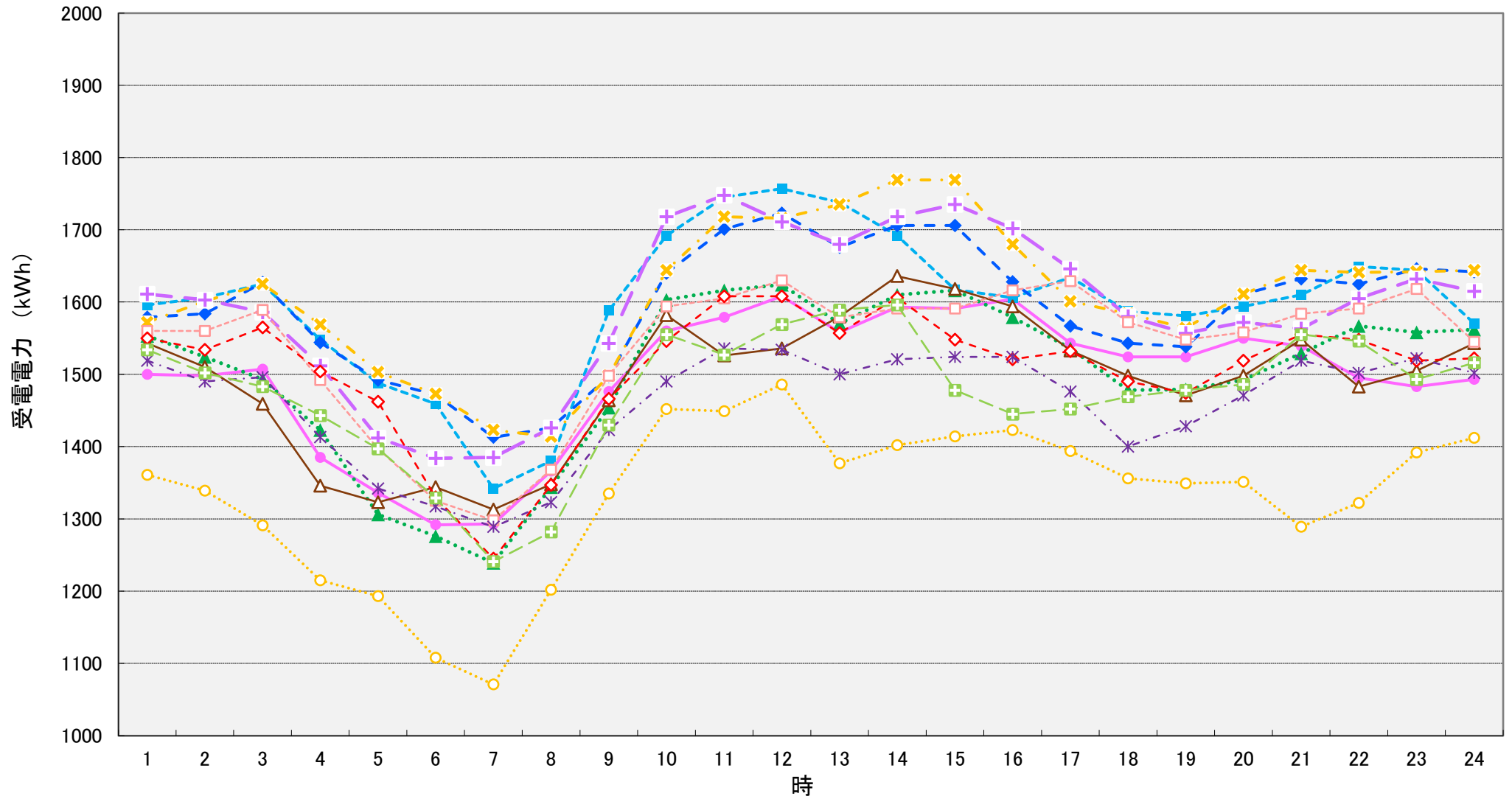
令和4年度 月別最大負荷日 負荷曲線 (アクアパル千曲)
