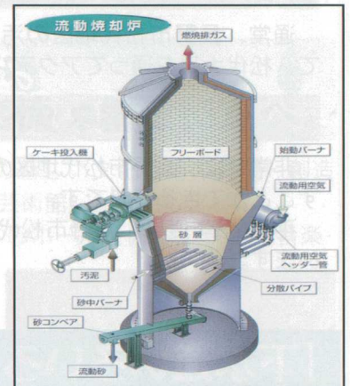
流動焼却炉本体
