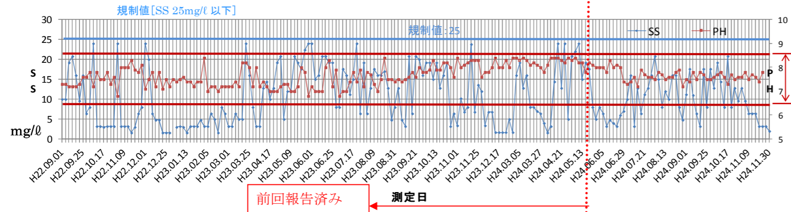
図 5.3.1 濁水処理後の放流水
