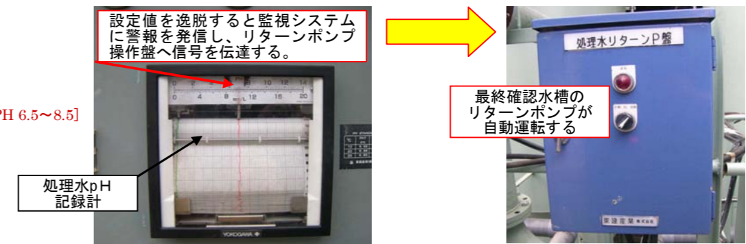
図 5.3.2 排出基準逸脱時の警報・自動返送機能
