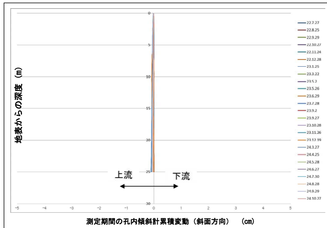
図 4.3.1 法面観測データの一例
