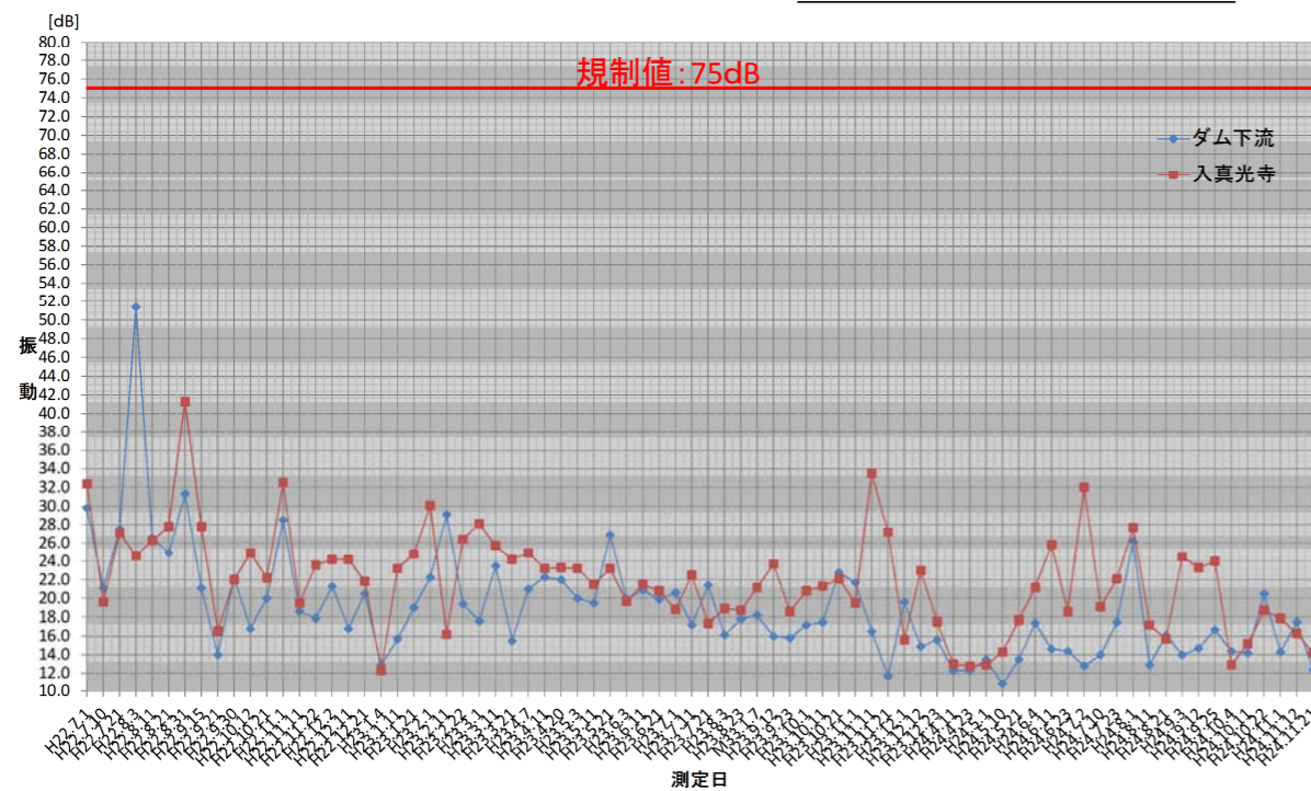
図 5.2.2 振動測定値グラフ
