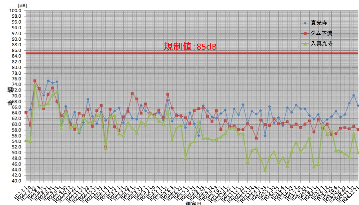
図 5.2.3 騒音測定値グラフ
